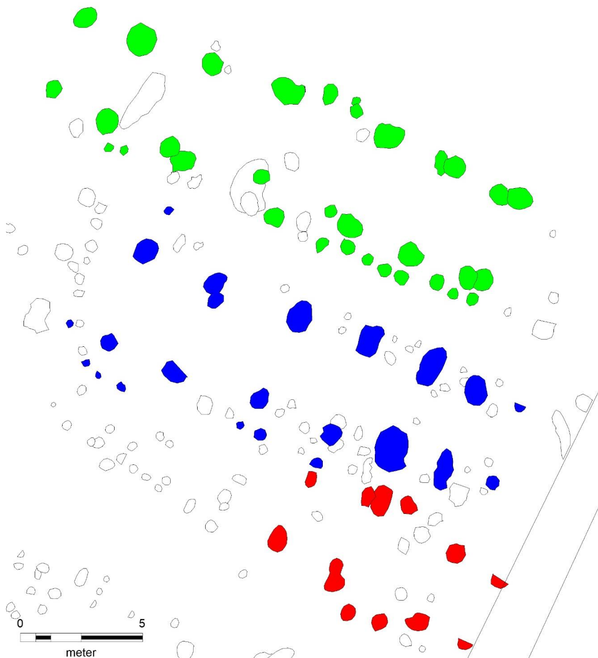
Figur 3. Plan med tagbærende stolper, indgangs- og vægstolper i hus A270 (grøn), hus A271 (blå) og hus A272 (rød) (© Nordjyllands Historiske Museum).
