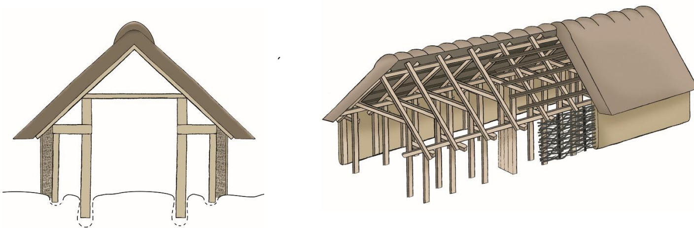
Figur 2: 3-skibet lanhus.
