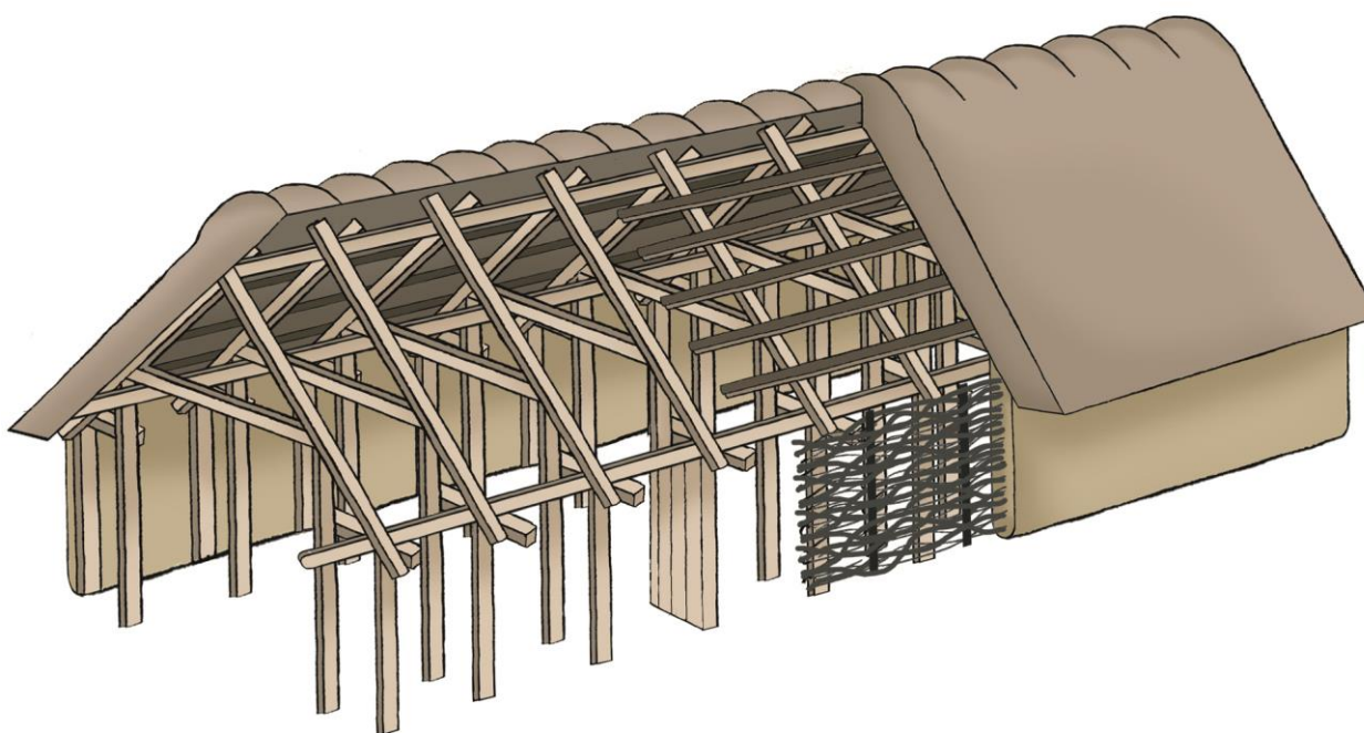
Figur 3 Perspektivtegning af konstruktionen af et treskibet bronzealderhus. To parallelle rækker af indre tagbærende stolper har båret husets tag, mens vægforløbet ofte har bestået af en let lerklinet feltvæg.
