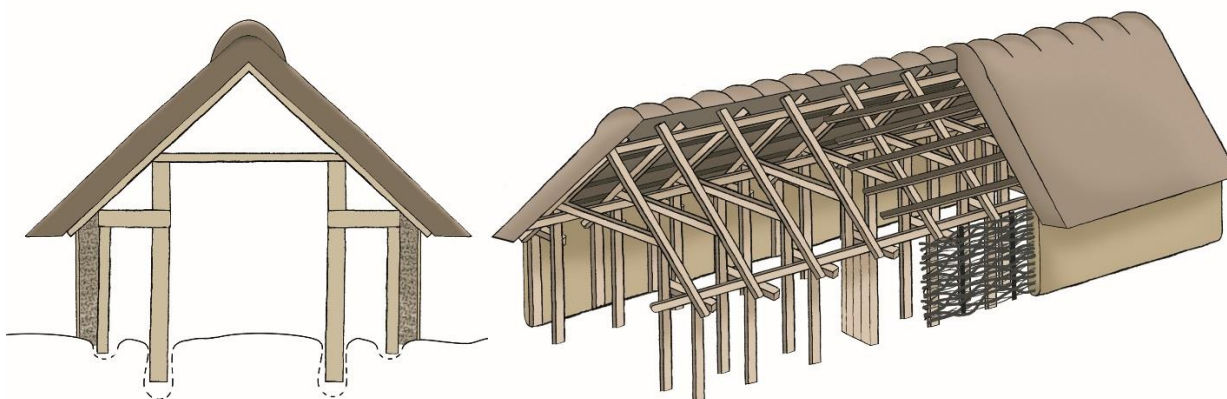
Figur 6: Hovedbygningen i gården fra yngre bronzealder er båret af to indre rækker af træstolper. Tilsammen danner de en treskibet konstruktion. Sådan byggedes husene igennem store dele af oldtiden, fra ældre bronzealder og ind i vikingetiden.
