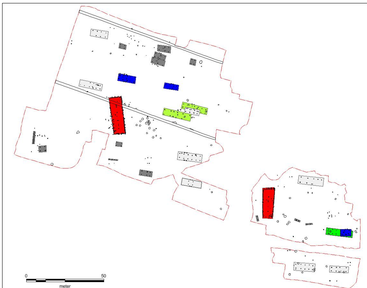
Figur 3. Udgravningsfeltet med alle oldtidshustomter markeret. Rød = de to store huse fra bondestenalderen. De øvrige farver er bygninger fra yngre bronzealder og førromersk jernalder. De mørkegrå er små udhuse.
