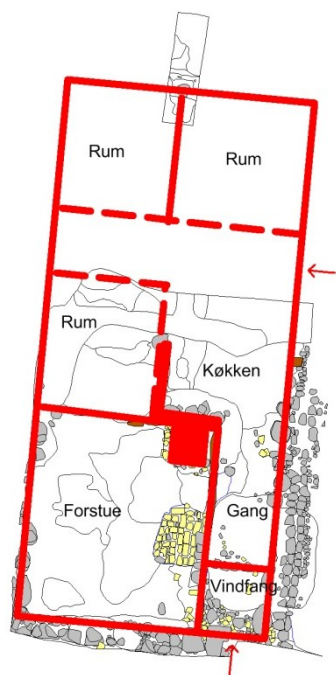
Figur 34. Et forslag til hvordan det vestlige beboelseshus omtrent var indrettet. Vindfanget var en sekundær indretning i huset.
