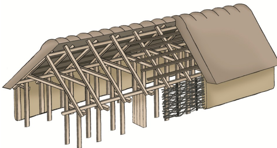
Figur 3 Rekonstruktionstegning af et treskibet oldtidshus, hvor husets tagbærende konstruktion bæres af to parallelle rækker af tagbærende stolper i husets indre.
