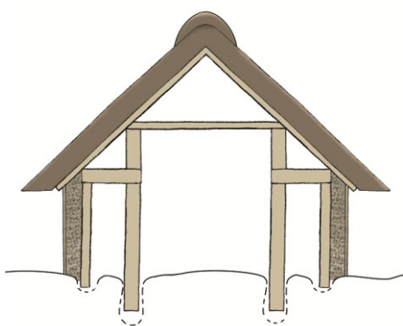
Figur 4 Tværsnit der afspejler opbygningen af den tagbærende konstruktion i et treskibet langhus.
