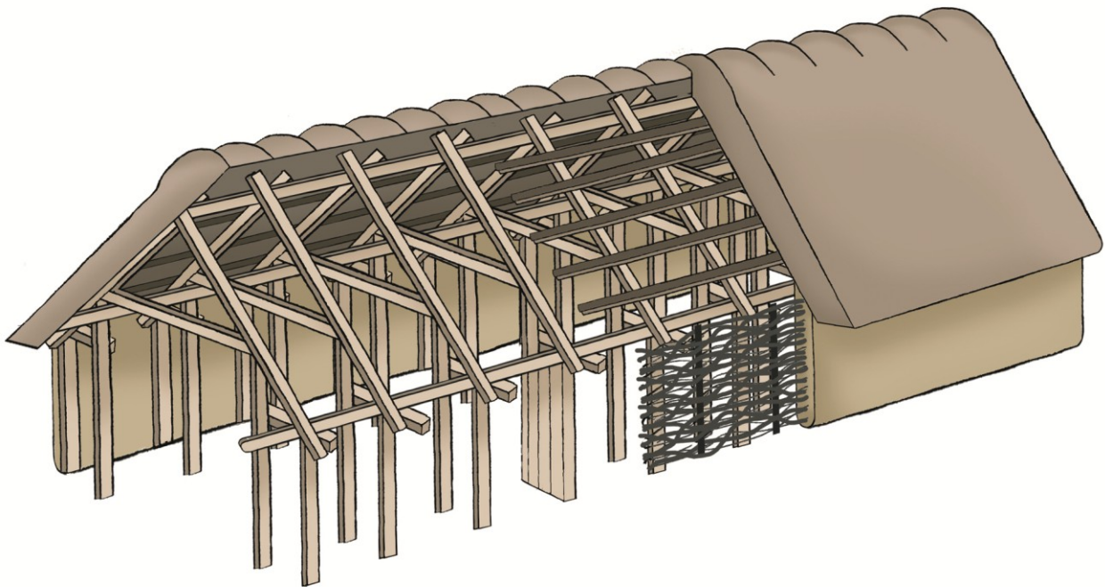
Figur 3. Rekonstruktionstegning af et treskibet oldtidshus, hvor husets tagbærende konstruktion bæres af to parallelle rækker af tagbærende stolper i husets indre. Ved Ellidshøj-bebyggelsen ser nogle af husenes vægge dog helt anderledes ud, med dybt funderede, tætstillede træplanker, i stedet for de lavere funderede fletvægge, der er illustreret her.
