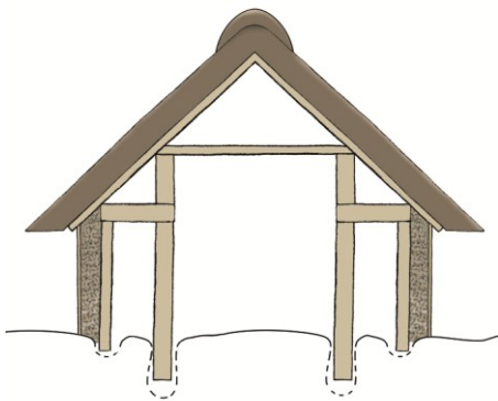
Figur 4. Tværsnit der afspejler opbygningen af den tagbærende konstruktion i de treskibede langhuse.
